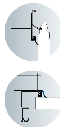
Thermische onderbreking
